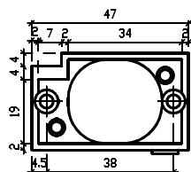
Widok z tyłu rozeta montażowa II
