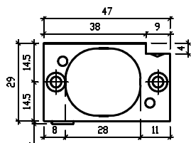
Widok z boku rozeta montażowa II
