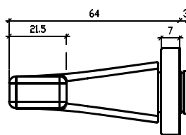
Widok z prawej strony klamka I
