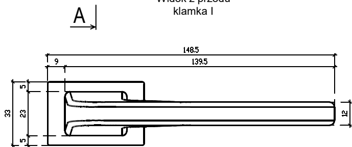
Widok z przodu klamka I
